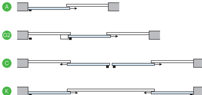
Pho 310 + 330 klassische Ausführung
