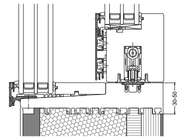
Pho 300 + 320 bodentiefe Verglasung
