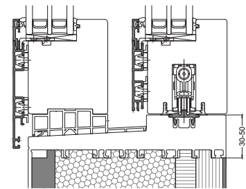
Pho 310 + 330 klassische Ausführung
